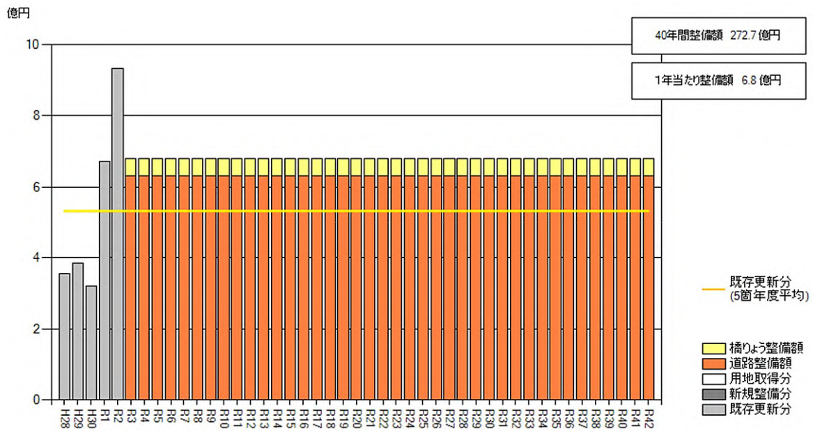
【図2-4-4】 今後40年間に要するインフラ施設の更新費用の将来推計（企業会計を除く。）】
