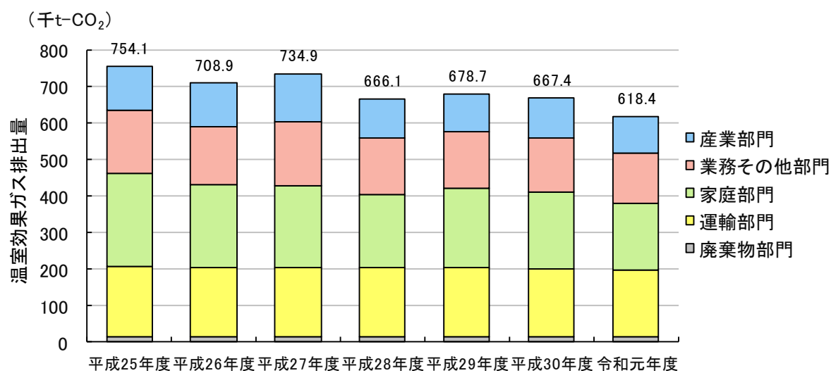
部門別温室効果ガス排出量の推移
